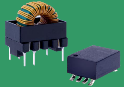
隔離（柵極驅動）變壓器
